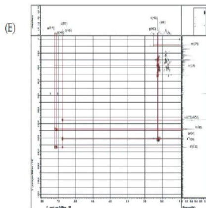
Gambar 5. Hasil spektra (A) ^1\text{H} -NMR, (B) ^{13}\text{C} -NMR, (C) COSY-NMR, (D)HMQC, (E) HMBC.
