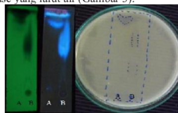
Gambar 3. Profil KLT fase larut \text{CHCl}_3 (A) dan fase larut air (B) dengan fase diam silika gel dan fase gerak kloroform:metanol:air (64:50:10 v/v) serta hasil uji bioautografi dengan bakteri S. aureus .
