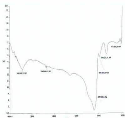
Gambar 4. Spektrum Infra Merah Isolat (dalam KBr).
