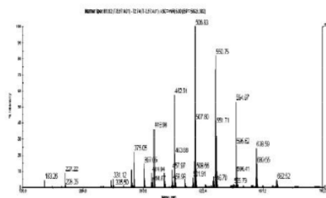
Gambar 6. Spektrum massa isolat dengan eluen metanol:air (90:10, v/v).
