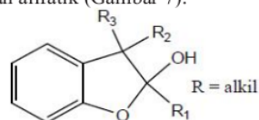
Gambar 7. Perkiraan struktur senyawa turunan benzofuran.
