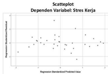
Gambar 3. Hasil Pengujian Heteroskedastisitas
