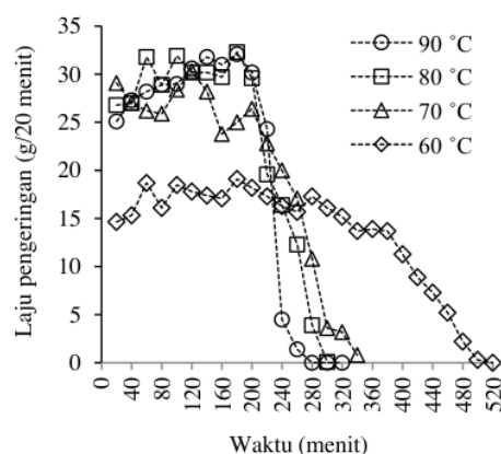
Gambar 4 Laju pengeringan vs waktu
