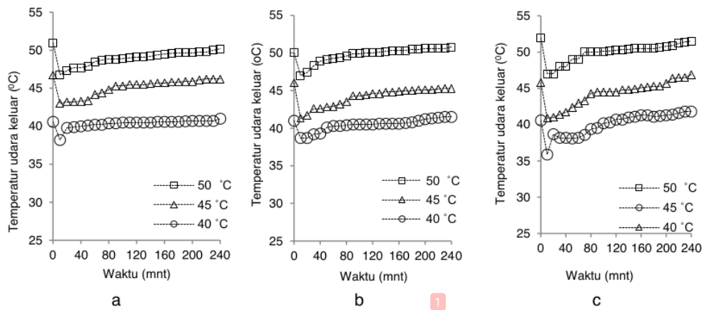
Gambar 6. Temperatur udara keluar untuk massa sampel (a). 200 gr, (b). 250 gr dan (c). 300 gr
