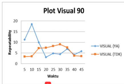
1 Gambar 1. Run Chart Repeatability Visual Pada Intensitas Suara 90 dBA
