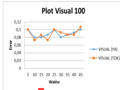
Gambar 8. Run Chart Error Visual Pada Intensitas Suara 100 dBA
