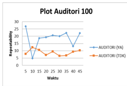
Gambar 4. Run Chart Repeatability Auditori Pada Intensitas Suara 100 dBA
