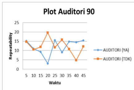
Gambar 3. Run Chart Repeatability Auditori Pada Intensitas Suara 90 dBA
