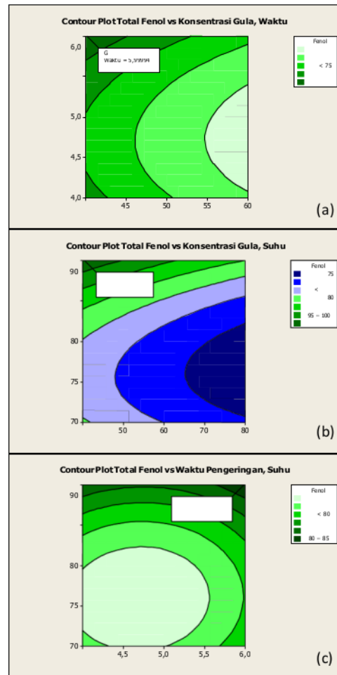
Gambar 2. Contour Plot Total Fenol vs Konsentrasi Gula dan Waktu Pengeringan (a), Contour Plot Total Fenol vs Konsentrasi Gula dan Suhu Pengeringan (b), Contour Plot Total Fenol vs Waktu dan Suhu Pengeringan (c)
