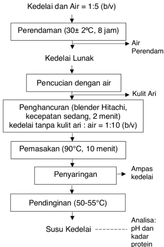
Gambar 1. Diagram alir pembuatan susu kedelai
