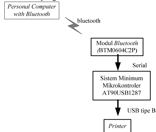
Gambar 3. Diagram blok sistem minimum dari mikrokontroler AT90USB1287
