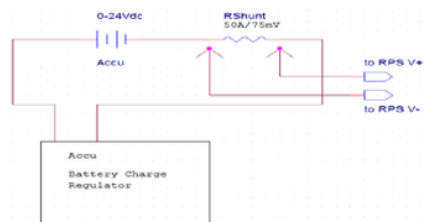
Gambar 10. Rangkaian Sensor Arus DC
