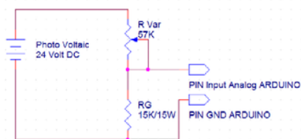
Gambar 11. Rangkaian Sensor Tegangan accu
