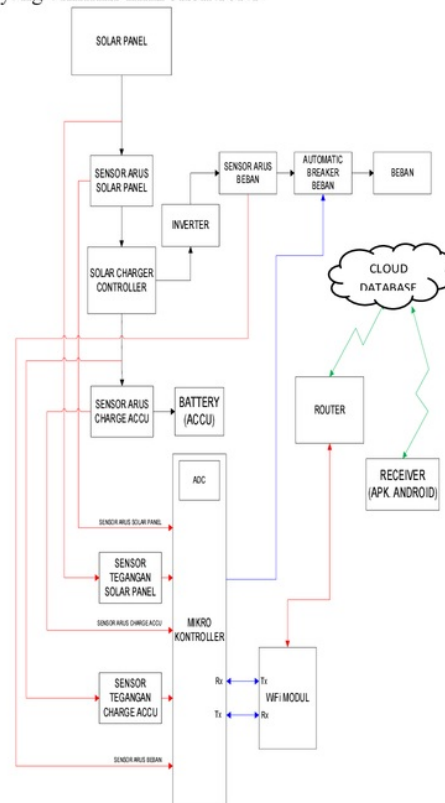
Gambar 9. Diagram Blok Alat
