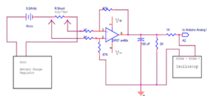
Gambar 12. RPS untuk Sensor Arus DC
