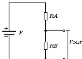
Gambar 5. Rangkaian pembagi tegangan
