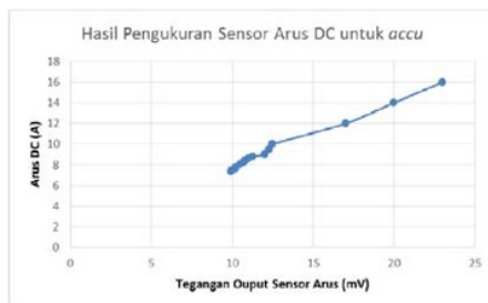
Gambar 14. Hasil Pengukuran Sensor Arus
