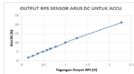
Gambar 15. Output RPS Sensor Arus DC untuk ACC
