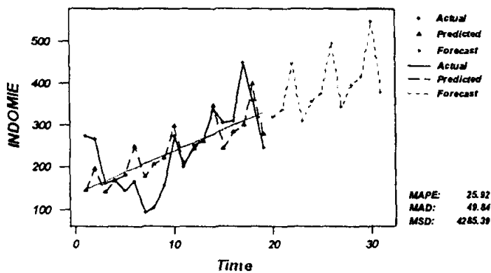
Decomposition Fit for INDOMIE
