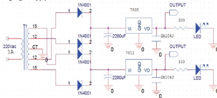
Gambar 8. Rangkaian skematik power supllly (Sumber: Dokumentasi pribadi, 13 Januari 2017)
