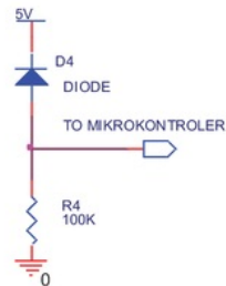
Gambar 7. Rangkaian sensor photodioda (Sumber: Dokumentasi pribadi, 13 Januari 2017)
