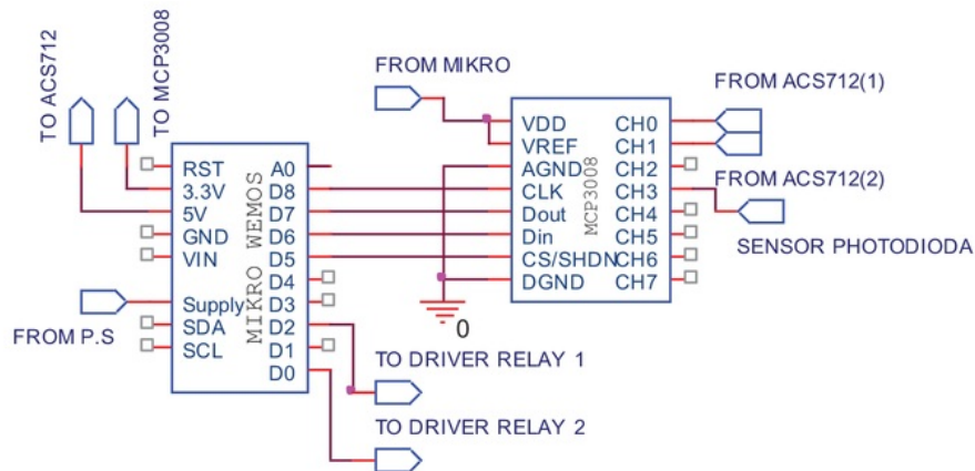
Mikrokontroler Wemos ini memiliki chipset ESP8266 yang berfungsi melakukan komunikasi secara wireless . Selain itu fungsi utama mikrokontroler berfungsi melakukan eksekusi terhadap data-data input yang berupa tegangan (analog) yang diolah oleh IC eksternal ADC.
