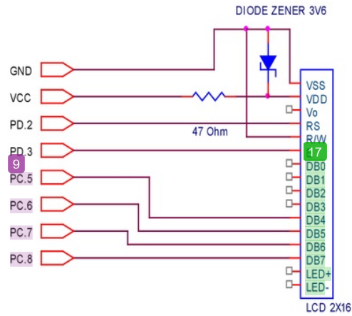
Gambar 10 Interface Receiver Mikrokontroler ATmega8535 Dengan LCD
