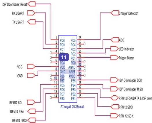
Gambar 9. Interface Mikrokontroler ATmega8L pada Slave
