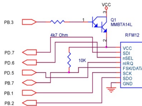
Gambar 11 Rangkaian Mikrokontroler ATmega8L Dengan Radio Frequency Module RFM12
