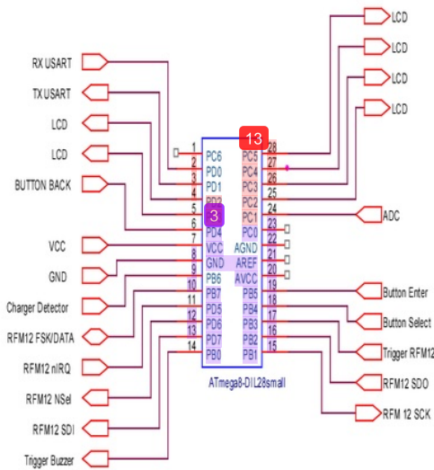
Gambar 8. Interface Mikrokontroler ATmega8L pada Master
