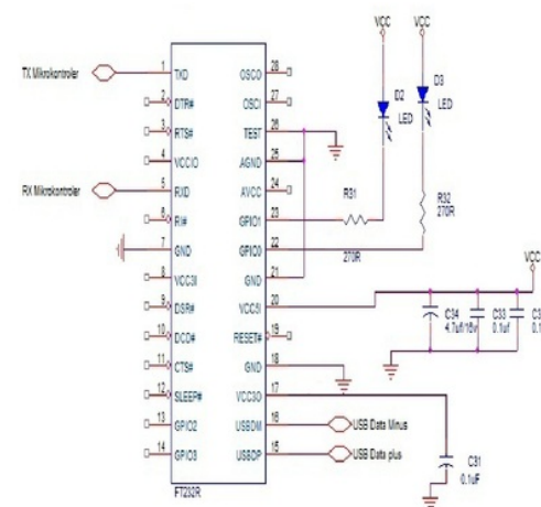
Gambar 7 gambar rangkaian FT232R
