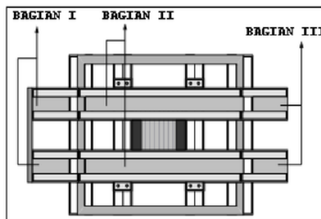
Gambar 6. Desain Kerangka Jembatan Timbang Tampak Atas
