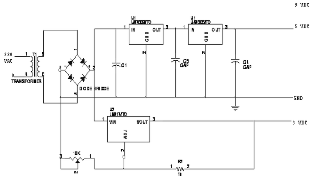
Gambar 11. Rangkaian Catu Daya
