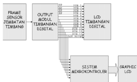
Gambar 5. Interkoneksi Sistem Jembatan Timbang
