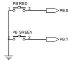
Gambar 8. Rangkaian Push Button
