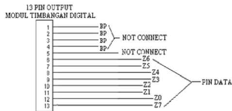
Gambar 7. Konfigurasi 13 Pin Output Modul Timbangan Digital
