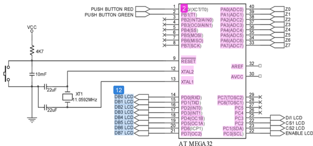
Gambar 10. Koneksi Rangkaian Mikrokontroler
