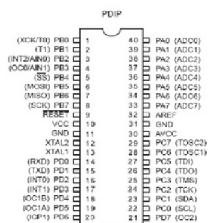
Gambar 2. Konfigurasi Pin ATmega32
