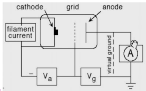
Gambar 1. Skema rangkaian percobaan Franck-Hertz
