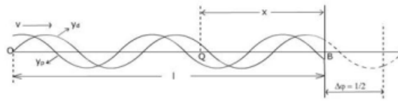
Gambar 5. Gelombang berdiri ujung terikat
