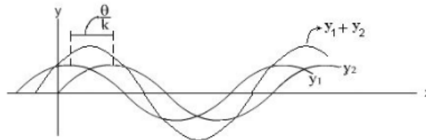
Gambar 4 Superposisi dua gelombang
