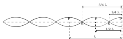
Gambar 8. Hasil interferensi
