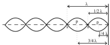
Gambar 6. Hasil interferensi
