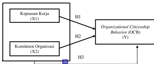
Gambar 1. Kerangka Penelitian
