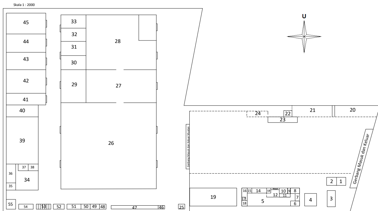
Gambar 2. Tata Letak PT. Menara Jaya Lestari Skala 1 : 2000
