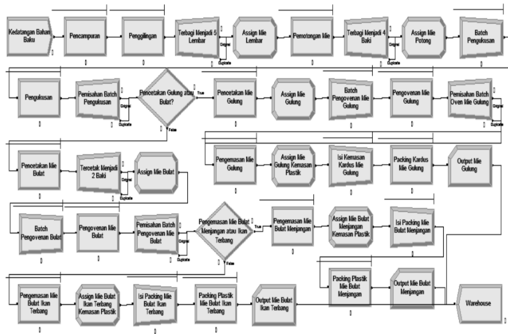
Gambar 2. Flowchart Proses pada Software Arena
