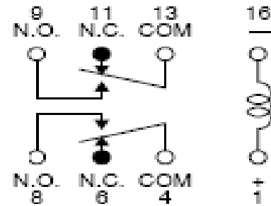
Gambar 16. Skema relay
