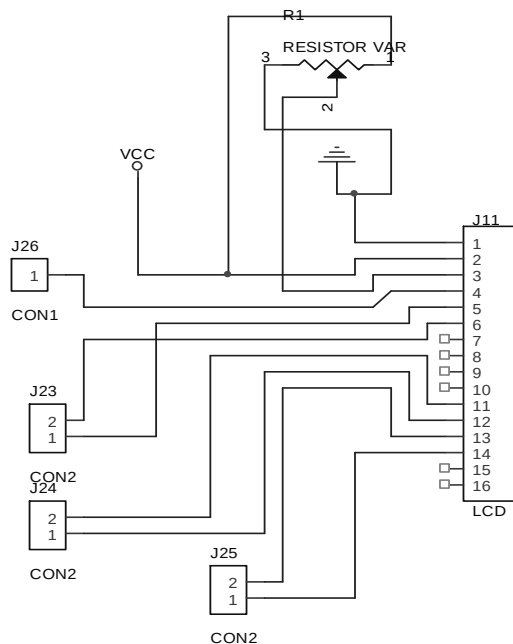
Gambar 21. Rangkaian LCD
