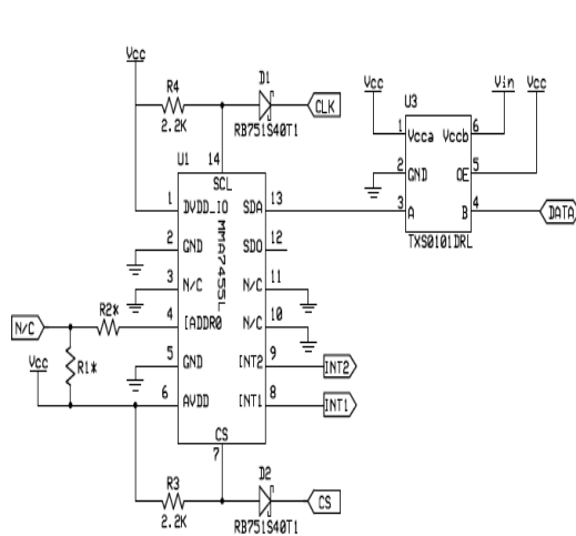
Gambar 18. Rangkaian acclerometer MMA 7745
