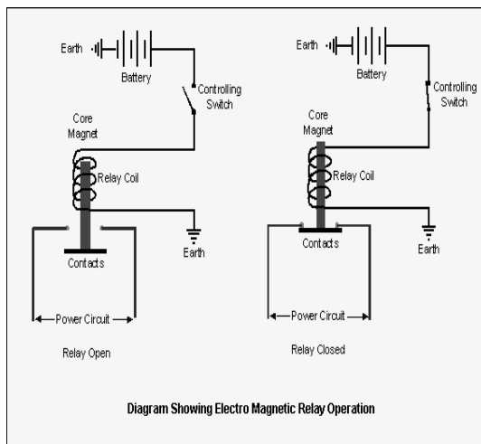
Gambar 15. Cara kerja relay
