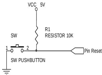
Gambar 5. Skematik rangkaian reset
