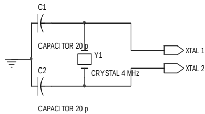
Gambar 4. Skematik rangkaian pembangkit sinyal
