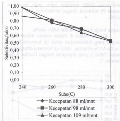
Gambar 5. Hubungan antara suhu terhadap selektivitas untuk katalis Cu-Zn-Al1/ \gamma -Al 2 O 3
