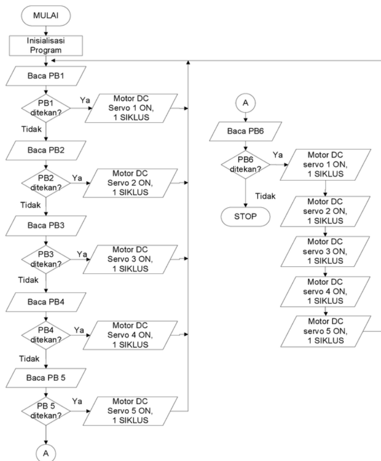
Gambar 10. Flowchart perangkat lunak pada mikrokontroler
