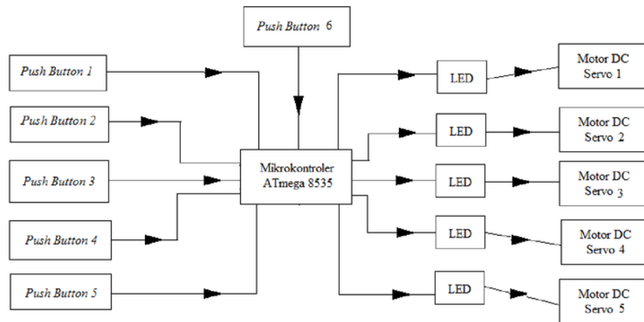
Gambar 8. Diagram blok alat
